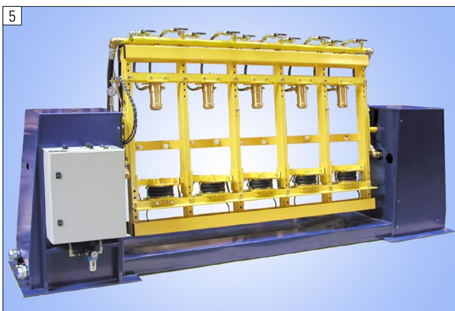
Rampe d'épreuve linéaire PTL-5 pour bouteilles domestiques
